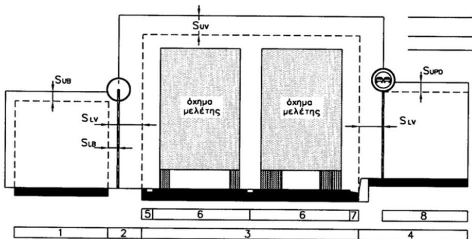
ΤΥΠΙΚΟ ΔΙΑΜΟΡΦΩΣΗΣ ΣΧΗΜΑΤΟΣ 7 (Τμήμα Α) - ΘΟΥΡΥΒΩΔΕΣ ΛΩΡΙΔΕΣ
